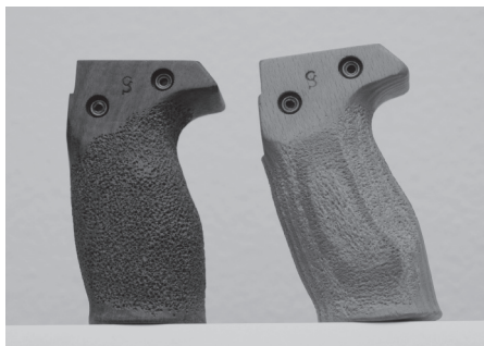
Bild 15: Standardgriffe 021101 und 021102 zu Stgw 57
