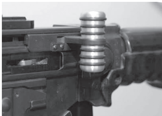
Bild 20: Ladegriff anatomisch zu Stgw 57
