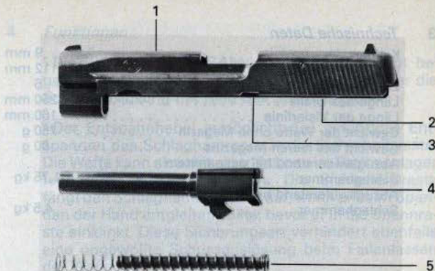
Bild 3 Beim Schuss beweglicher Teil
